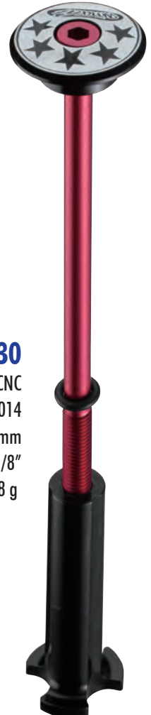
RS-2315 Material:AL6061 CNC Bolt : AL2014 Length : 210-270mm Size : 1-1/8" / 1.5" Weight : 72 g
